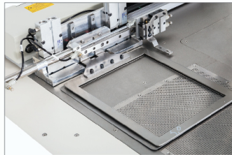
侧滑装置 Side slop device
